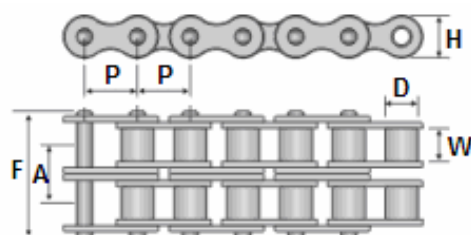
Corrente de transmissão dupla Norma AMERICANA ASA
