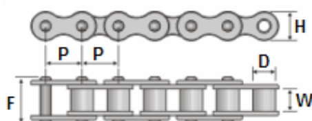
Corrente de transmissão simples Norma AMERICANA ASA
